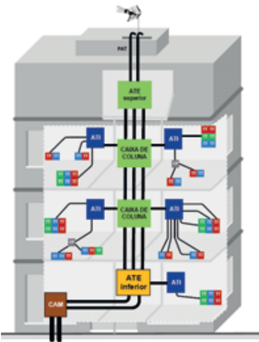
Esquemas da rede colectiva e individual, fonte Manual ITED 4ª Edição.
