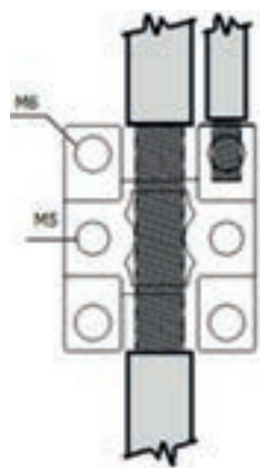
SECÇÃO DERIVADA Cabo Rígido: 4 - 16mm 2 Cabo Flexível: 4 - 10mm 2
